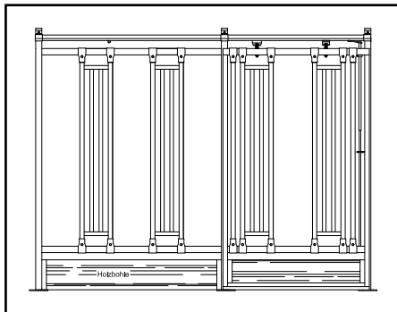
Vorderfront mit Sicherheits-Durchfressgitter & Schiebetür (Preis ab 733,- € + MwSt.)
