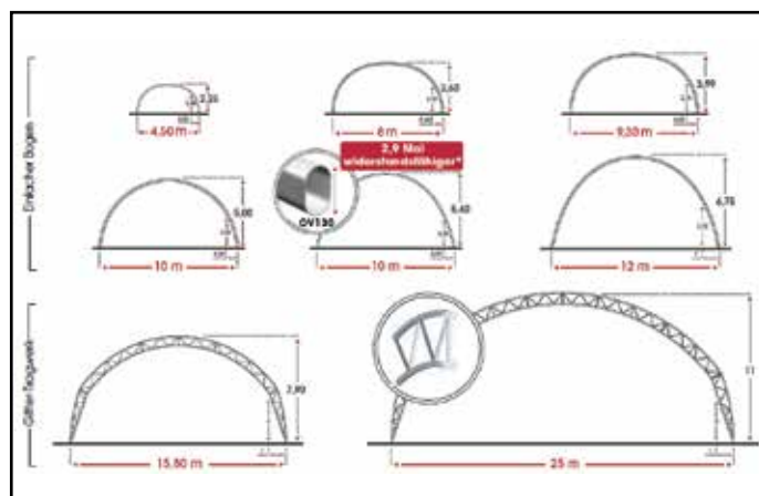
Maschinenhalle 12,00 m breit x 6,75 m hoch
