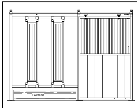
Vorderfront mit Sicherheits-Durchfressgitter & Schiebetür Holz/Gitter (Preis ab 733,- € + MwSt.)
