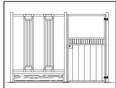
Vorderfront mit Sicherheits-Durchfressgitter & halbhoher Drehtür (Preis ab 700,- € + MwSt.)
